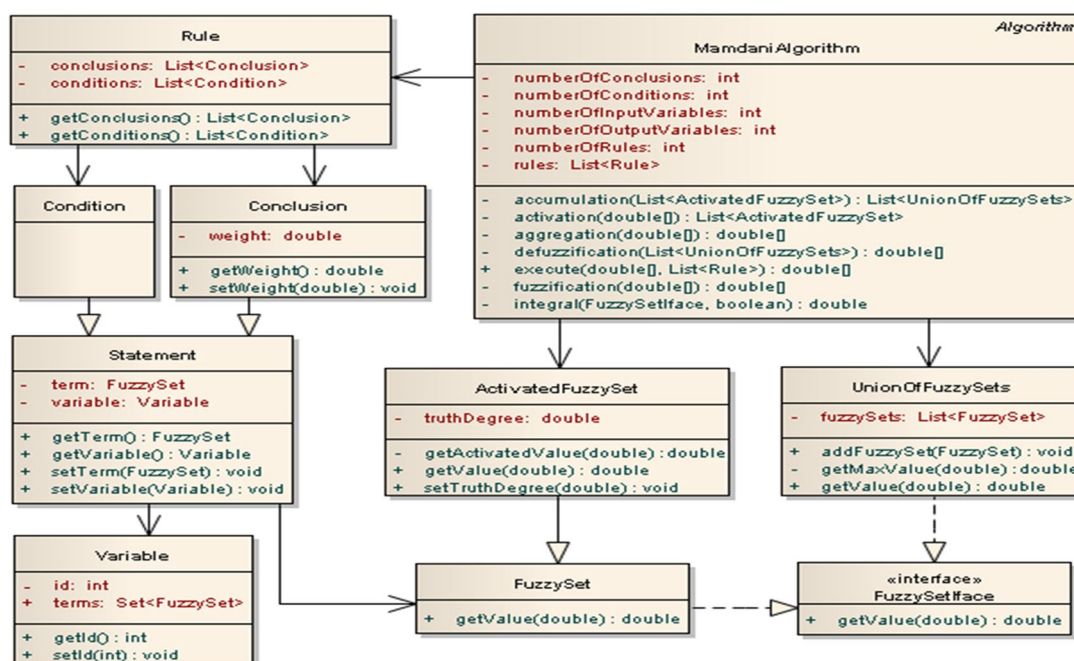
Рис. 4. Диаграмма классов реализации алгоритма Мамдани [2, 3].
