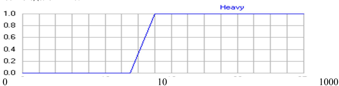
рис 1 График функции принадлежности \mu(x) для нечеткого множества В [1]
