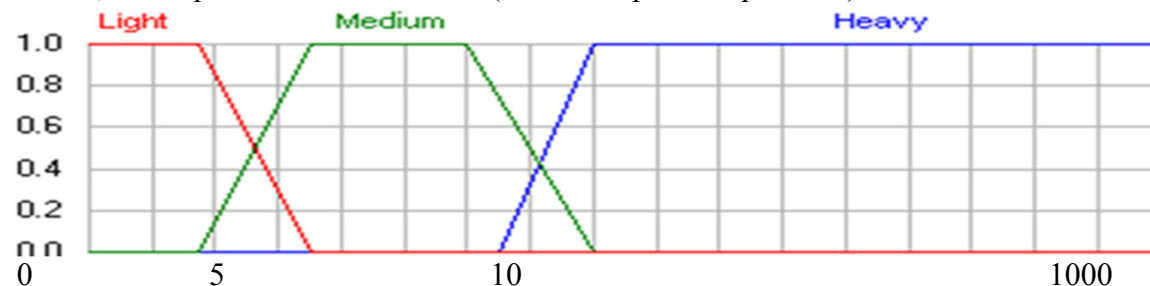
Рис. 2. Графики функций принадлежности значений лингвистической переменной «количество адресов» [1, 2].
